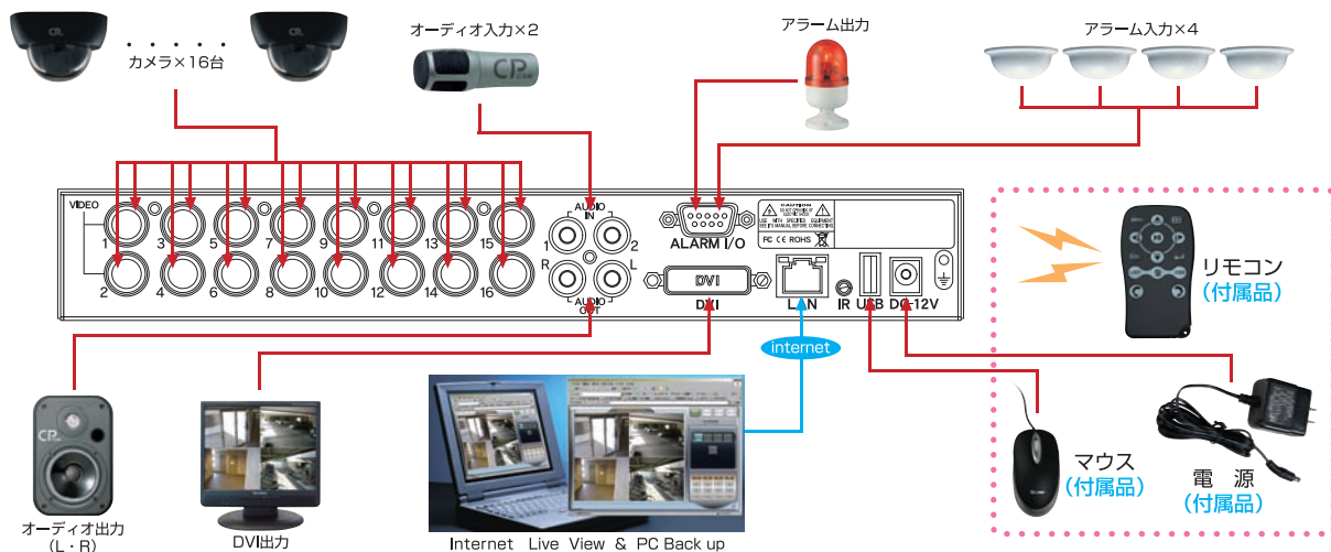
■システム構成図
